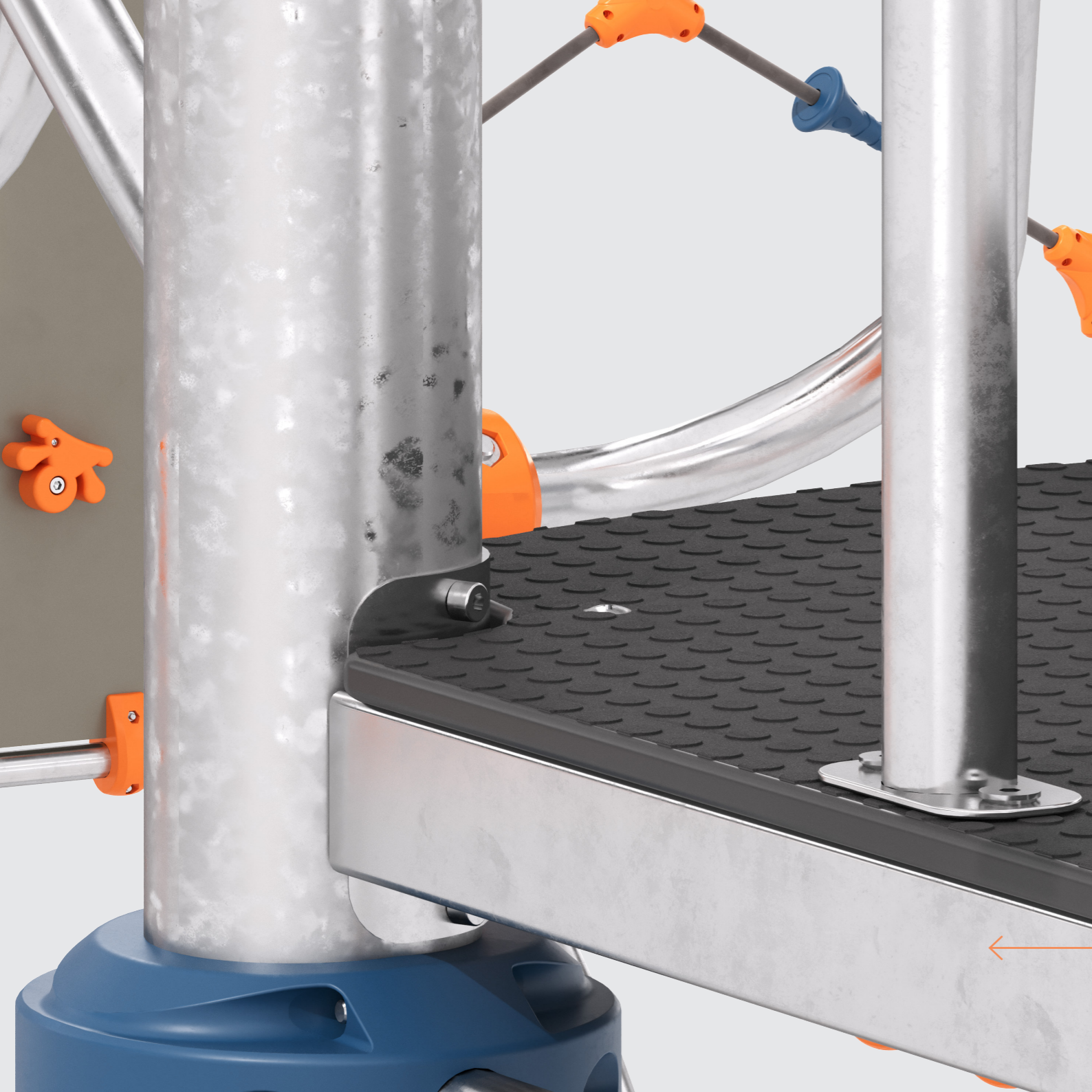
17 ТРУБЫ Ø108 ММ И ДУ25 Оцинкованная и нержавеющая сталь Трубы из оцинкованной и нержавеющей стали. Покраска по заказу.
