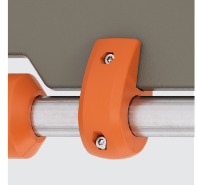
22 СОЕДИНИТЕЛЬ «HDPE-ТРУБА» Стеклонаполненный полиамид Предназначен для крепления HDPE-пластика (15 мм) к трубе ДУ25.
