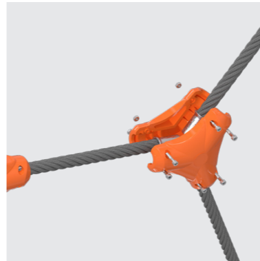
18 СОЕДИНИТЕЛЬ ДЛЯ КАНАТА Полиамид (нейлон) 6 (РА6) Предназначен для соединения трех канатов Ø16 мм.
