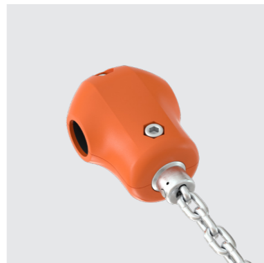
07 Т-ОБРАЗНЫЙ СОЕДИНИТЕЛЬ Стеклонаполненный полиамид Предназначен для соединения трубы ДУ25 с ДУ25 или с цепью.
