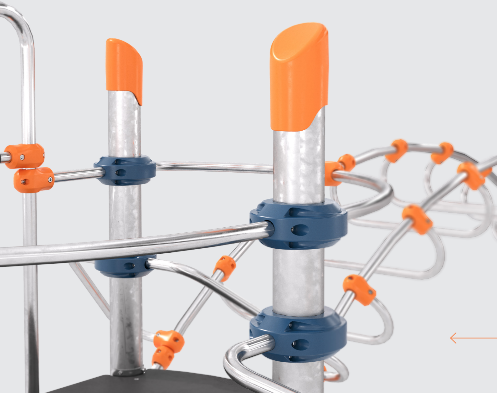
24 СОЕДИНИТЕЛЬ «ТРУБА-КАНАТ» Стеклонаполненный полиамид Предназначен для соединения трубы ДУ25 с канатом Ø16 мм.
